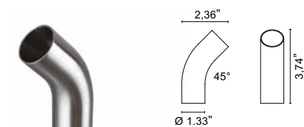
45° expanding bend Curva de sujeción de 45
