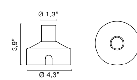
Draining box Encofrado drenante
