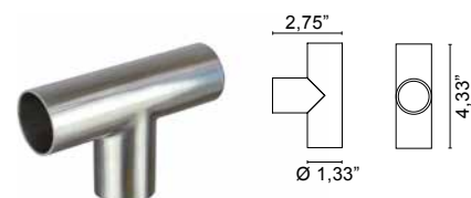
T joint expanding bend Junta en T con mandril
