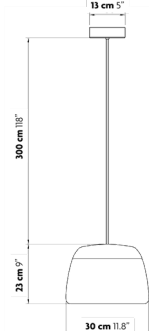
Ice Absolut 30 Pendant
