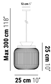
O'R Big Pendant
