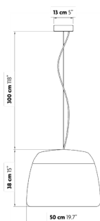
Ice Absolut 50 Pendant
