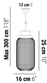
O'R Slim Pendant
